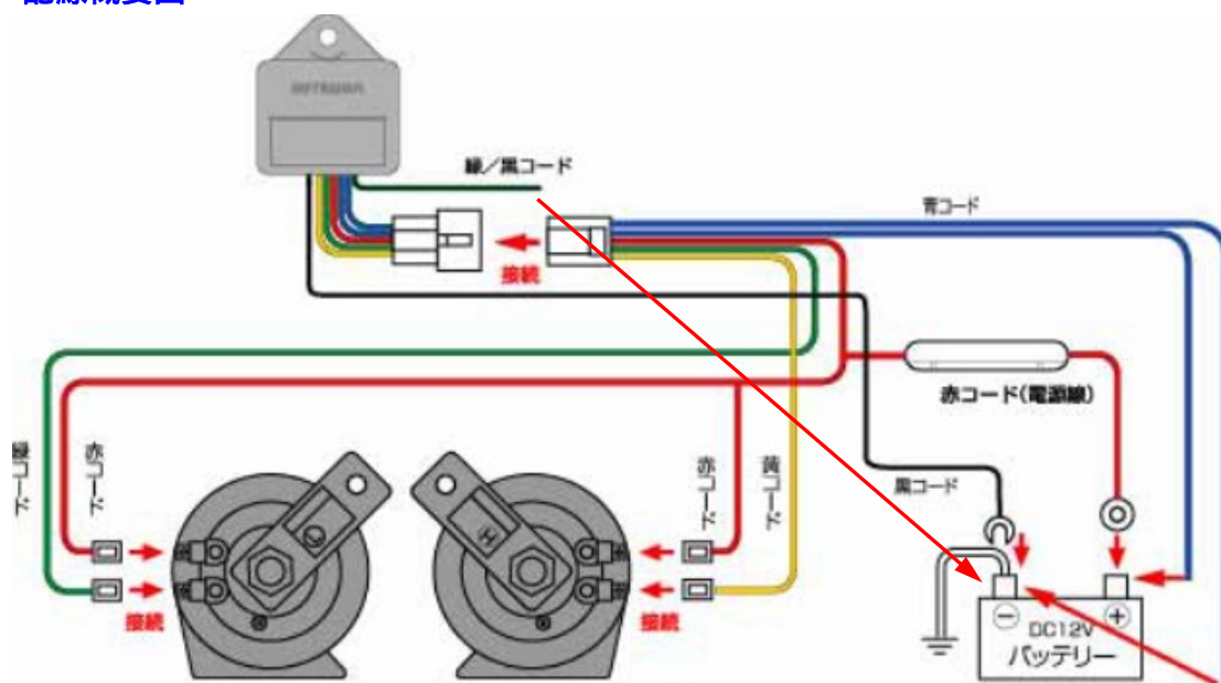
配線概要図
