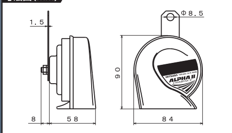
寸法図 (mm)
